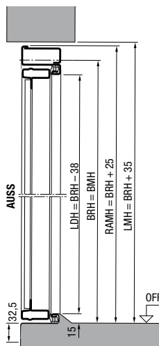
Przekrój pionowy drzwi z progiem
